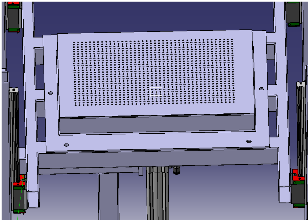
Слика 6.9 Вакуумска плоча намонтирана на њено постоље
