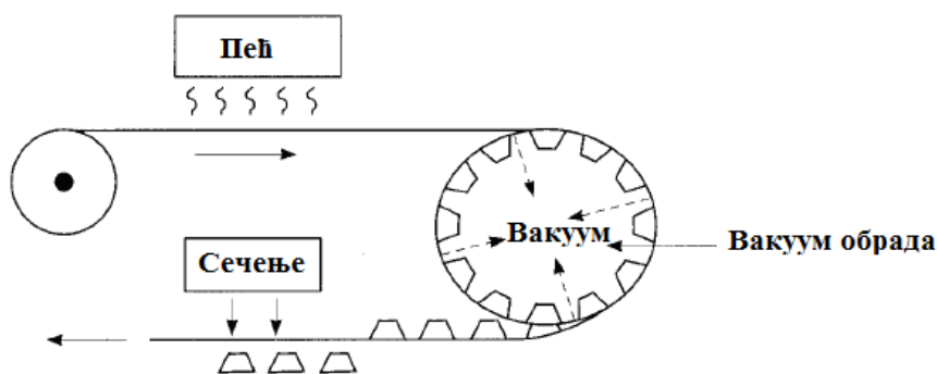
а) Термообликовање са континуалним дозирањем фолије
