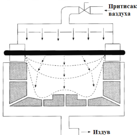
Слика 3.2 Обликовање притиском [8]
