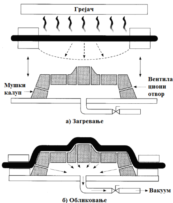
Слика 3.6 Вакуумско обликовање са предразвлачењем [8]
