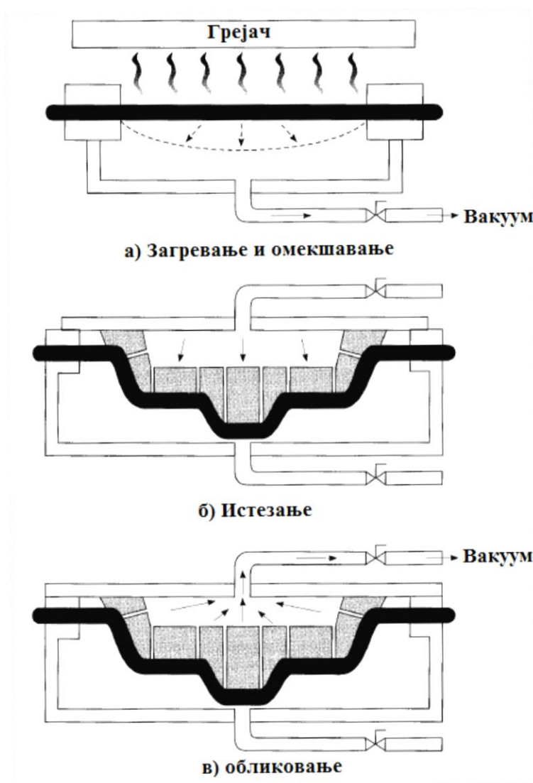
Слика 3.8 Топло обликовање у калупу са вакуумским предобликовањем [8]
