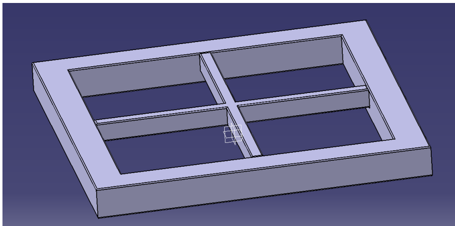
Слика 6.5 Постоље машине за вакуум термообликовање
