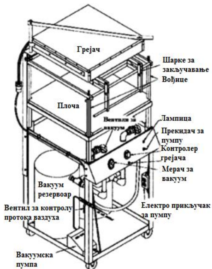
Слика 6.1 Склоп машине за вакуум – термообликовање [1]
