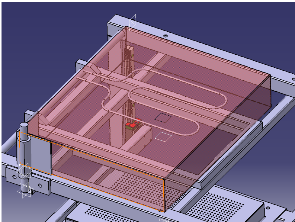
Слика 6.11 Хауба грејача са грејачем на окретном механизму
