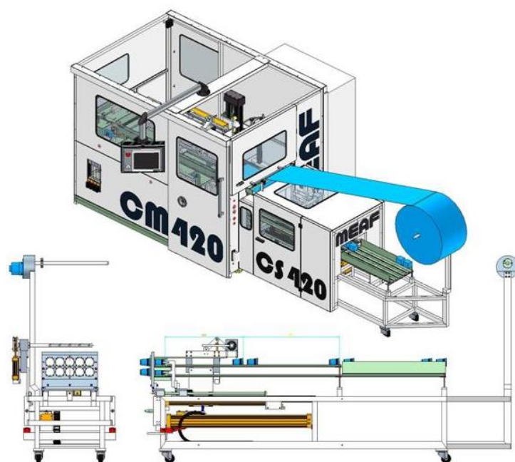
Слика 5.7 Изометриски поглед моделиране машине CM420 [6]
