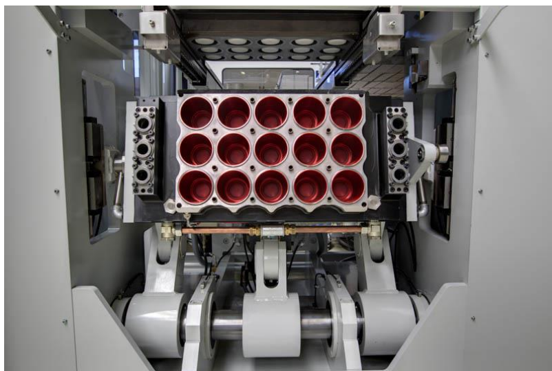
Слика 5.3 Изглед калупа за термоформинг на машини KMS600 [6]
