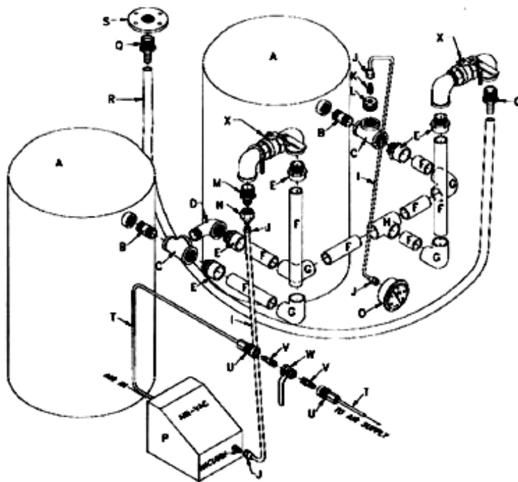
Слика 6.4 Склоп вакуумске инсталације [1]
