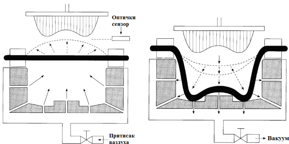
Слика 3.4 Прва фаза обликовања [8]
