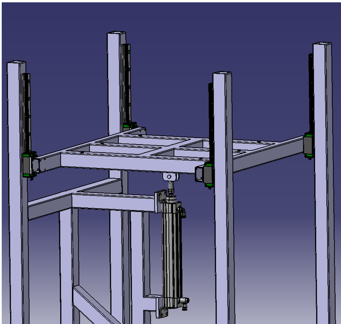
Слика 6.8 Линеарне вођице монтиране заједно са постољем алата на вертикалне стубове машине
