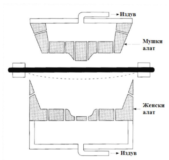
Слика 3.7 Обликовање помоћу дводелног алата [8]
