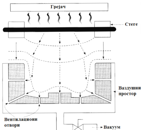
Слика 3.1 Вакуумско обликовање [8]
