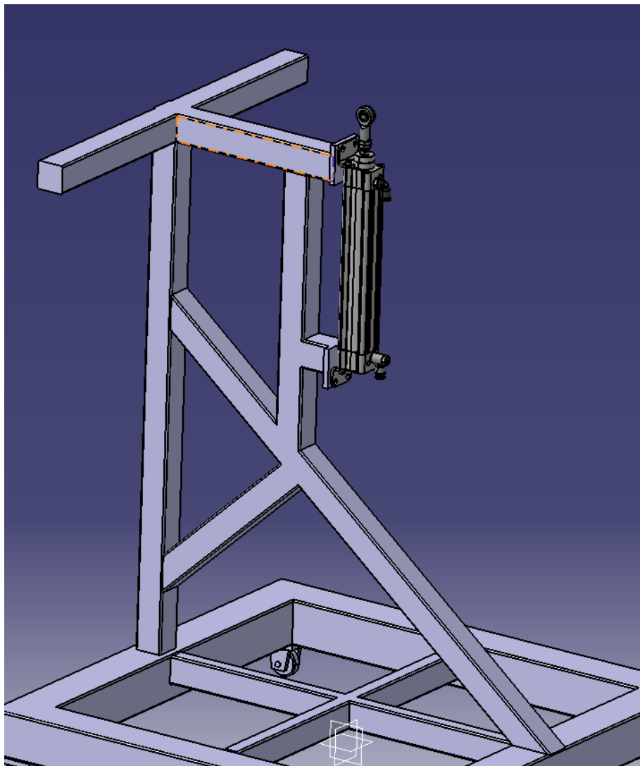
Слика 6.7 Пнеуматски цилиндар монтиран на конструкциону решетку
