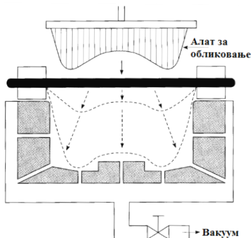
Слика 3.3 Обликовање помоћу обликача [8]
