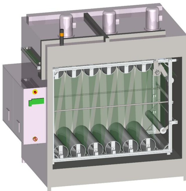
Слика 5.9 Унутрашњи изглед предгрејне коморе [6]
