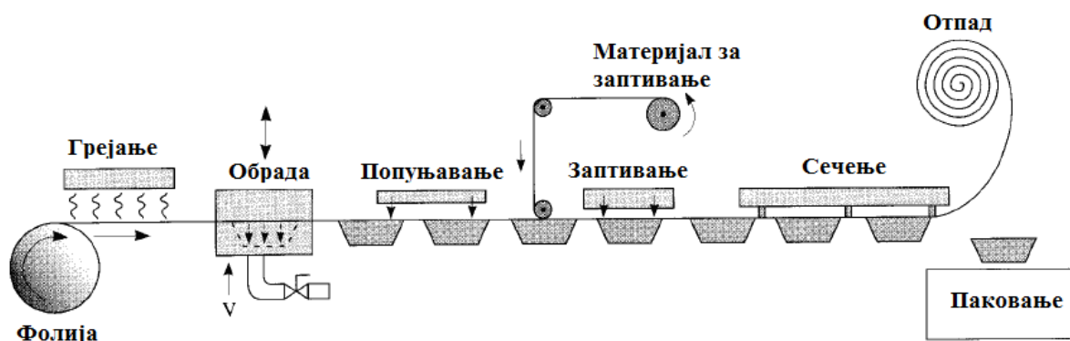
Слика 3.16 Пример континуалног топлог обликовања [8]
