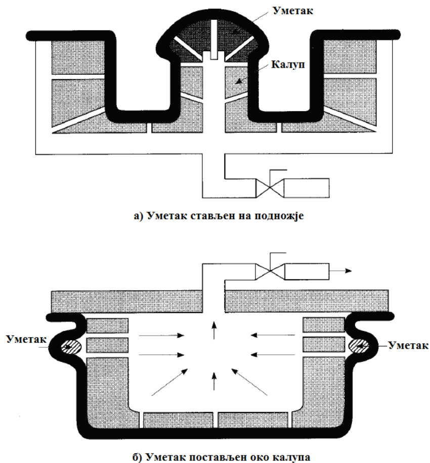
Слика 3.15 Пример сложенијег дела добијеног помоћу уметака [8]
