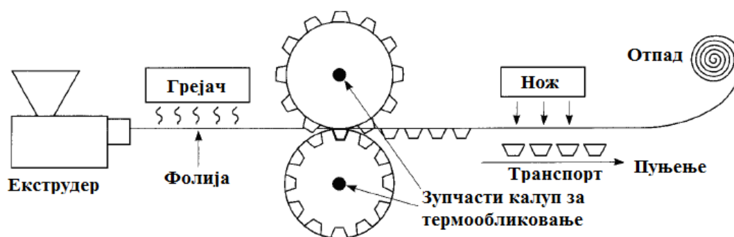
б) Екструзионо дозирање са зупчастим калупом за термообликовање
