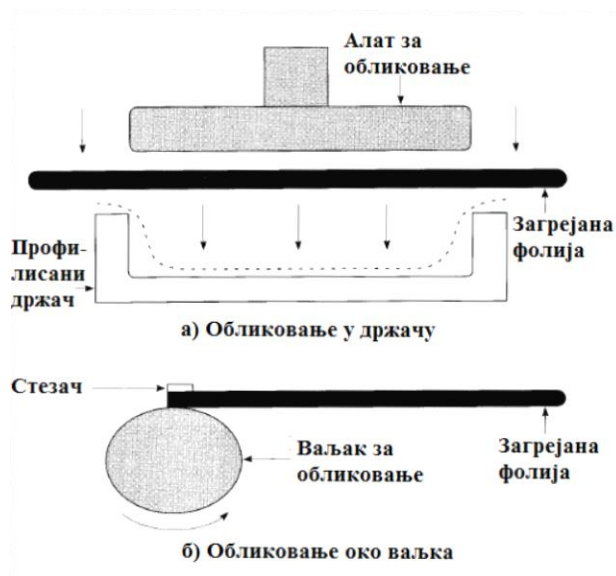
Слика 3.9 Механичко топло обликовање [8]
