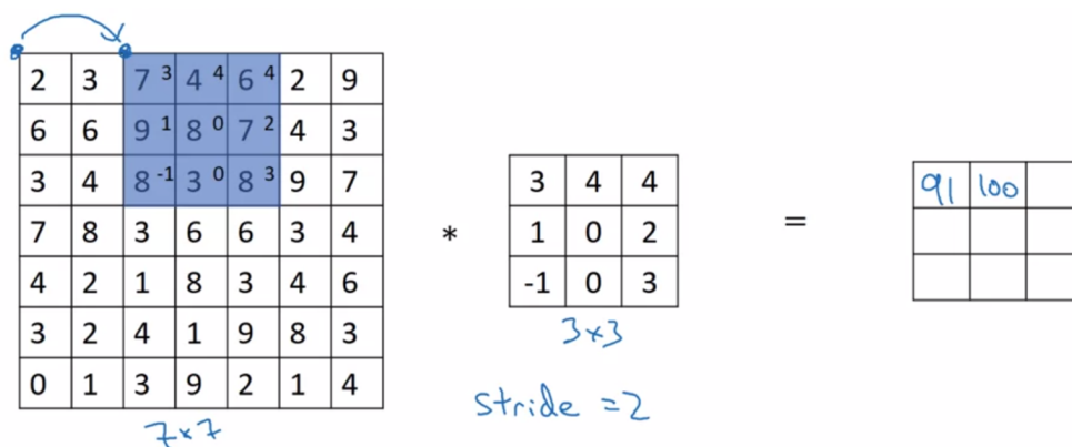
Слика 16: Конволуција са већим кораком исечка
