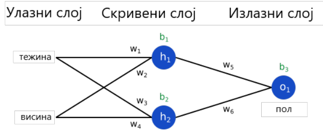
Слика 10: Тежине веза и прагови активације у вештачкој неуронској мрежи
