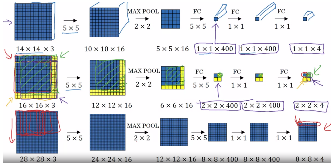
Слика 23: Детекција над сликама већих димензија
