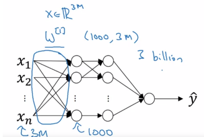
Слика 12: Превелика величина података на улазу у мрежу
