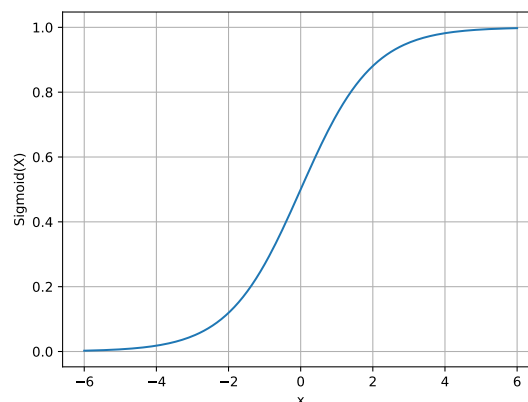
Слика 7: Сигмоидна функција
