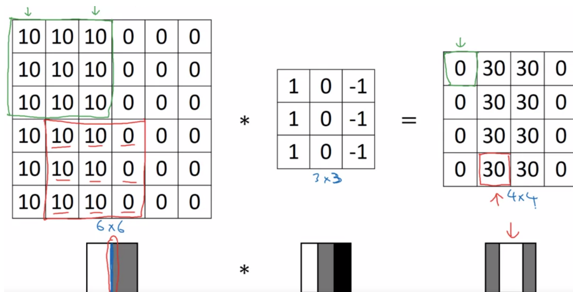
Слика 15: Вертикална ивица, прелаз светло-у-тамно
