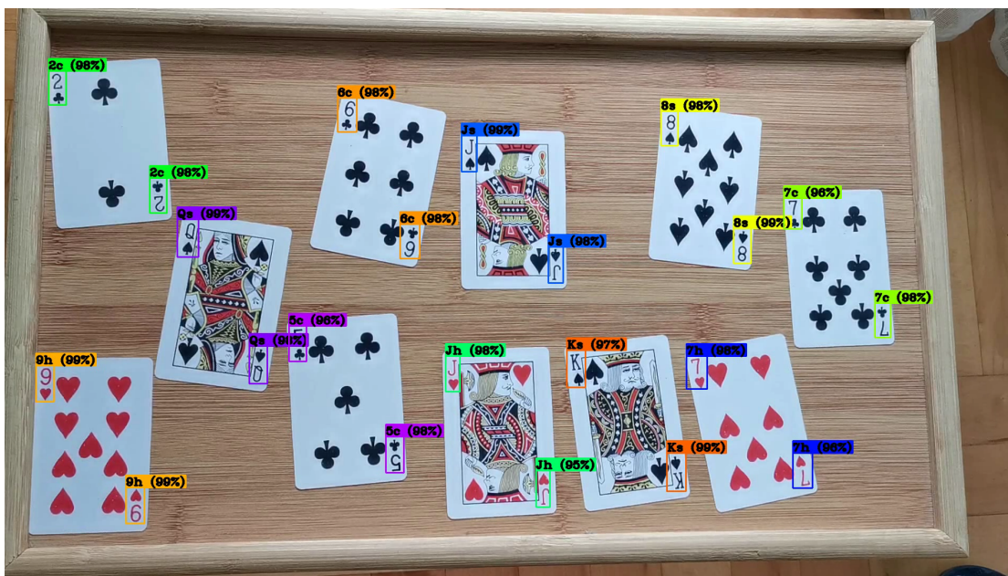
Слика 31: Тестирање над видеом
