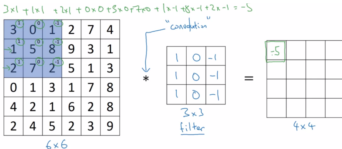
Слика 13: Операција конволуције
