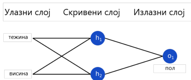
Слика 9: Вештачка неуронска мрежа која треба да се тренира
