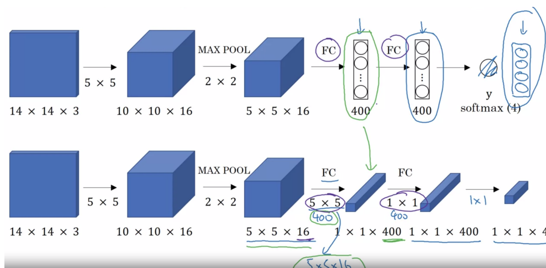
Слика 22: Имплементација клизних прозора применом конволуцијских мрежа
