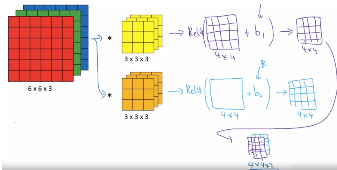
Слика 18: Пример слоја конволуцијске неуронске мреже
