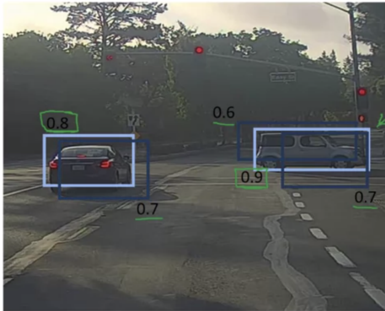
Слика 26: Више граничних оквира око истог објекта
