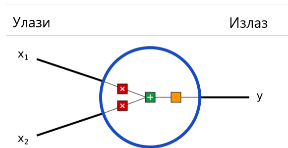
Слика 6: Неурон
