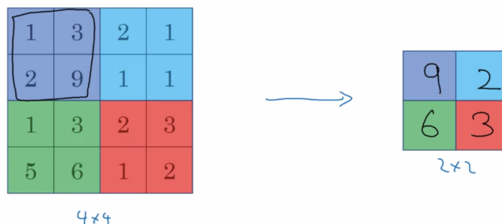
Слика 19: Max pooling
