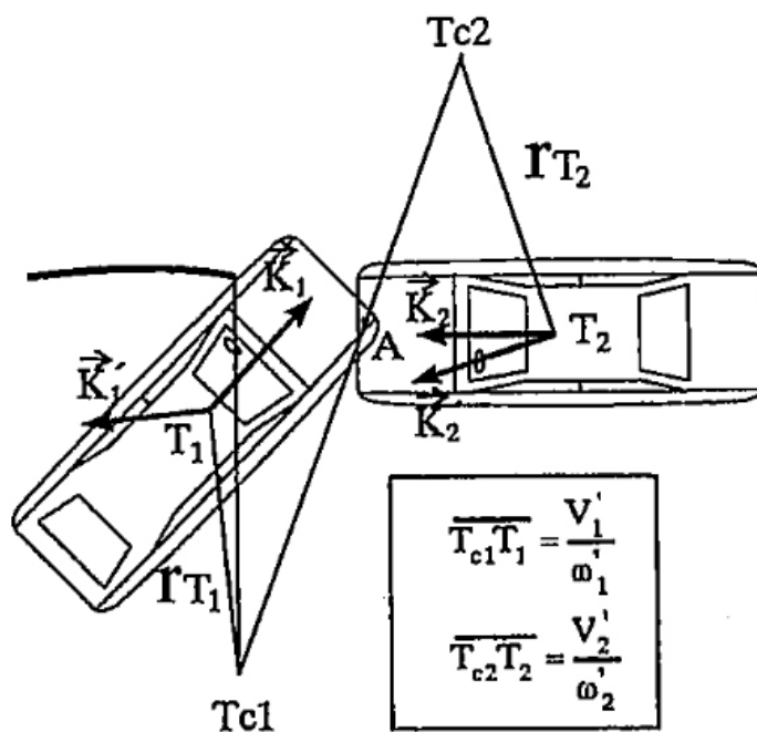
Слика 4. 11. Утврђивање тренутних полови и положаја вектора количина кретања аутомобила непосредно након судара, применом једначина Маркарда
