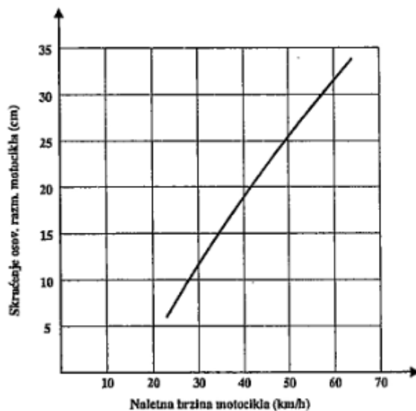
Слика 4. 19. Скраћење осовинског размака мотоцикла у зависности од сударне брзине
