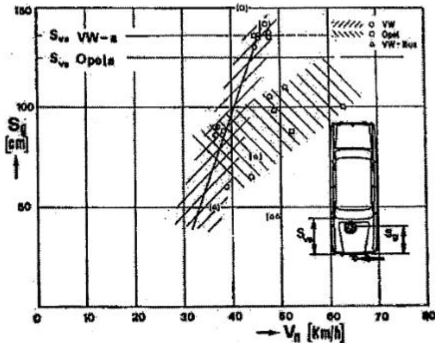
Слика 4. 16. Зависност сударне брзине од места удубљења ударом главе пешака
