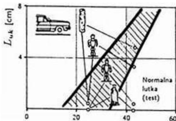
Слика 4. 18. Зависност између сударне брзине и дубине удубљења
