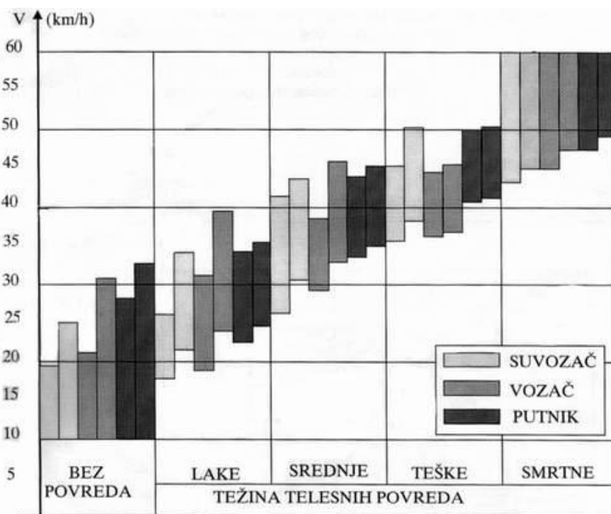
Слика 4. 15. Зависност сударне брзине и тежине телесних повреда [5]
