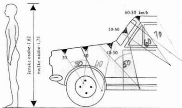
Слика 4. 17. Контактна места главе пешака у зависности од сударне брзине [5]
