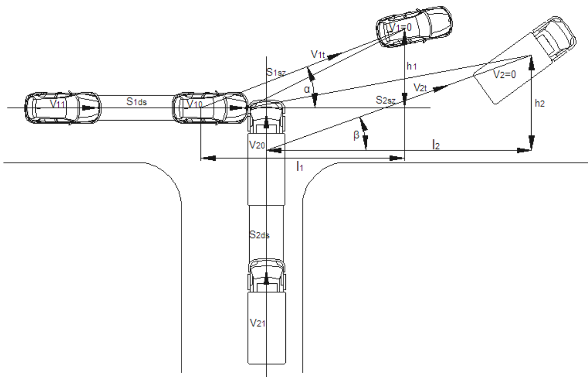
Слика 4. 5. Утврђивање брзине код чеono-бочних судара [1]
