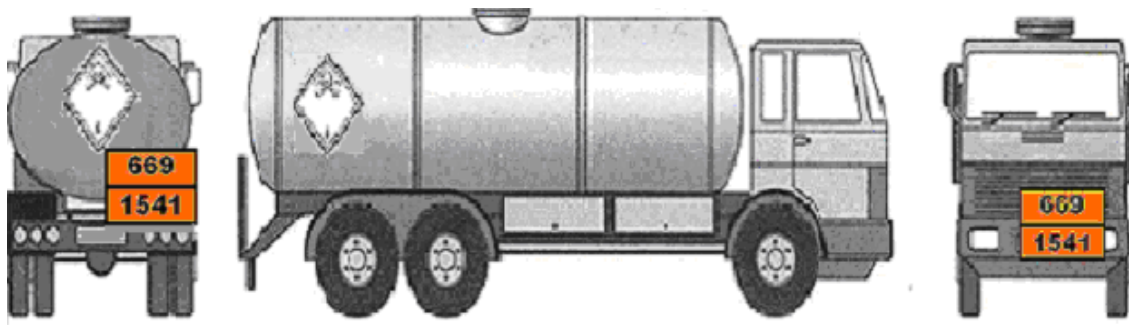
Слика број. 5. Возило- цистерна са изградњом без комора у коме се превози АЦЕТОН-ЦИЈАНХИДРИД СТАБИЛИЗОВАН
