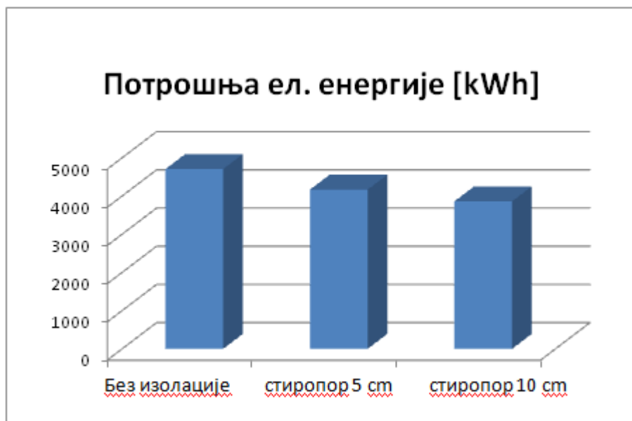
График 3. Количина утрoшене ел. енергије за грејање објекта
