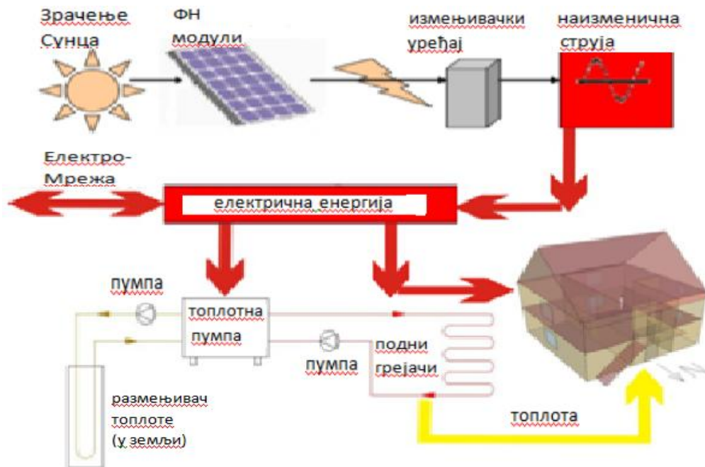
Слика 2. Принцип добијања и употребе ел. енергије у систему
