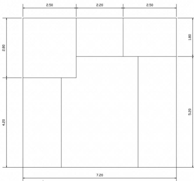
Слика 8. Димензије просторија објекта
